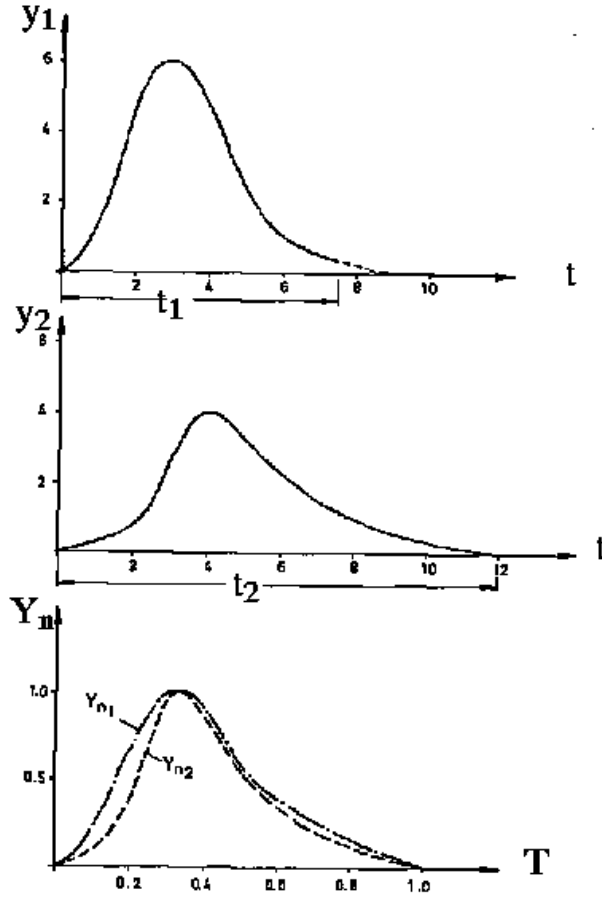
FIG 5: Normalisation of Parameters
